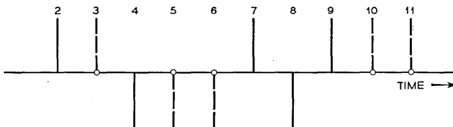
(d) DICODE TRANSMISSION (a)+(c)
