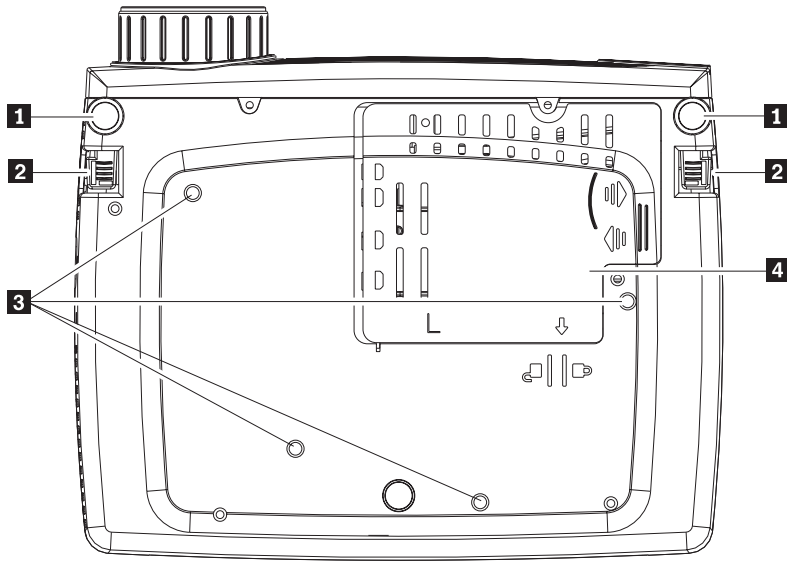
Slika 1-6. Pogled na dno projektora
