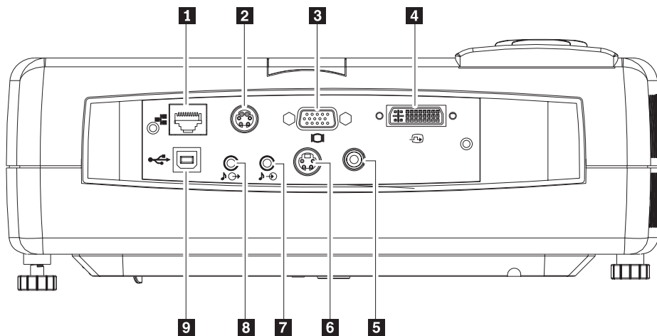
Slika 1-5. Pogled na stražnji dio projektora
