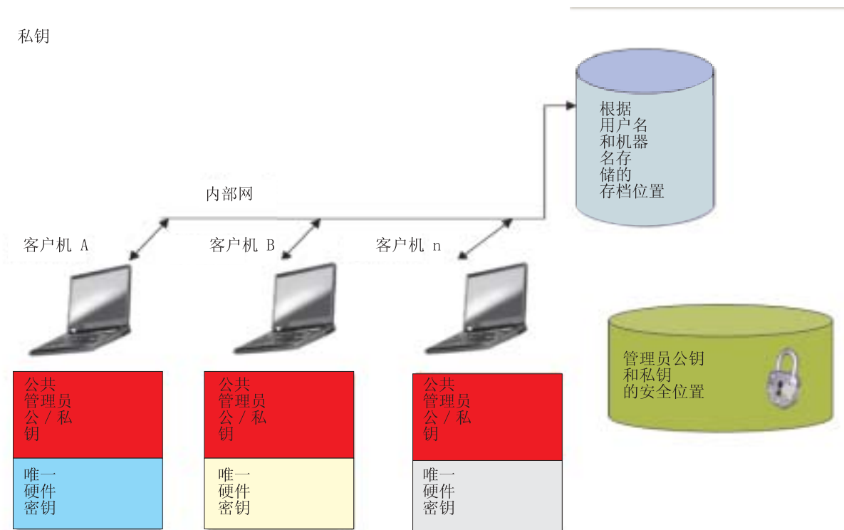
图 16. IBM 客户端安全系统的主要组件。
